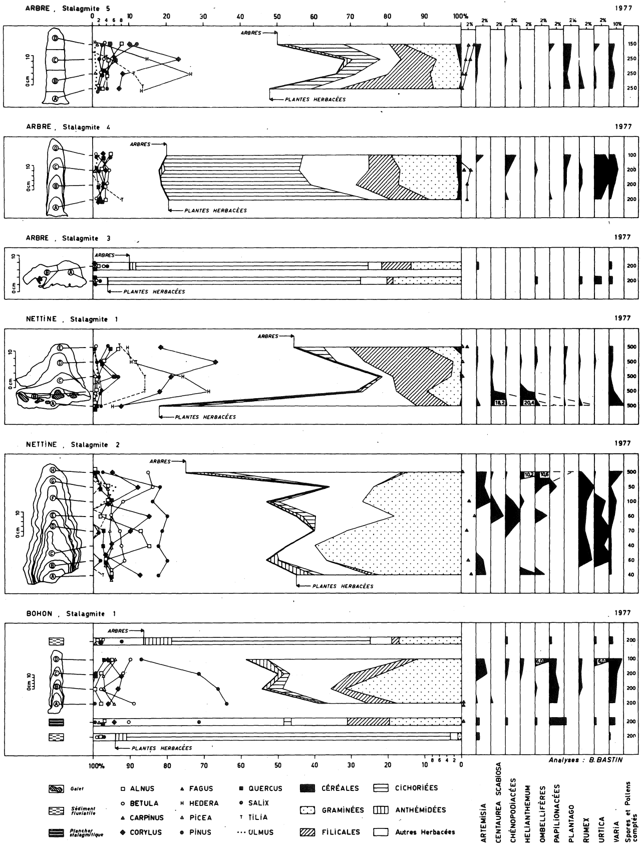
Figure 1.- Diagrammes polliniques obtenus dans six stalagmites prélevées dans trois grottes belges.
